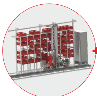
Αποθήκευση κιβωτίων με μεταφορικές ταινίες
